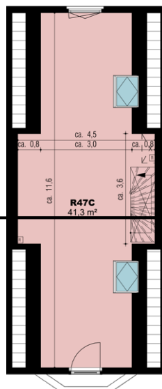
Derde verdieping
