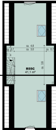
Derde verdieping
