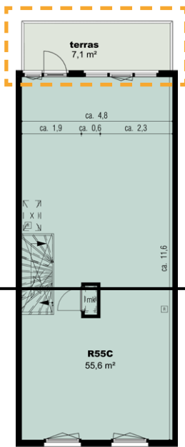
Tweede verdieping
