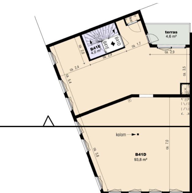
Tweede verdieping
