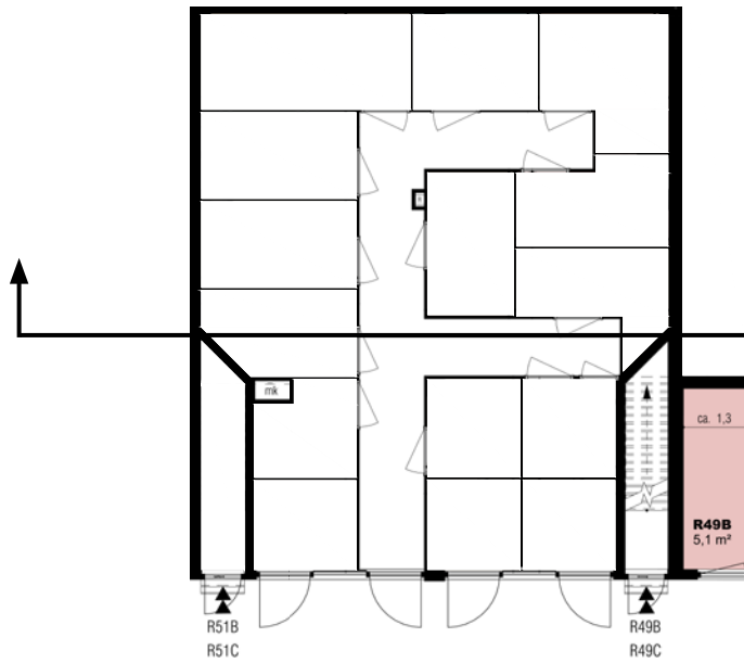
Begane grond
