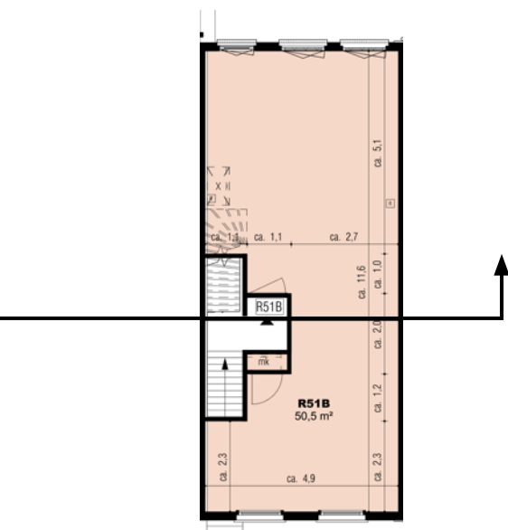
Eerste verdieping
