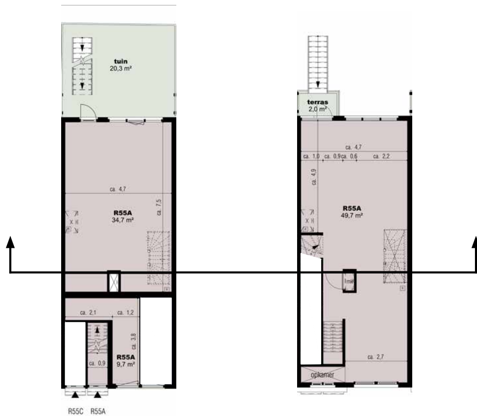
Souterrain
